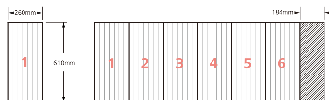
CSDR7 間口1820mmのシェルフ1段にCSDR7を6枚設置した場合 積載トレイ枚数: 42枚
